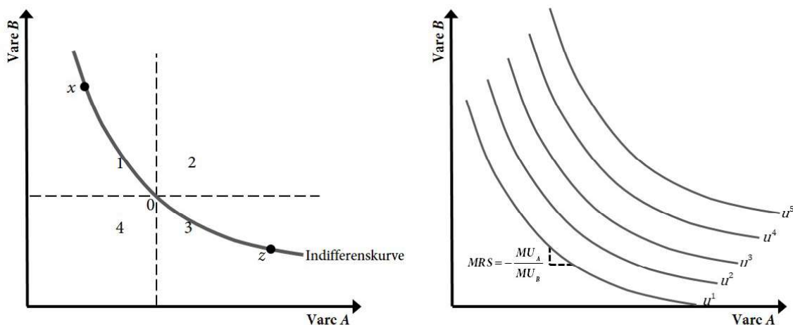
Figur 5a,b. Indifferenskurver
